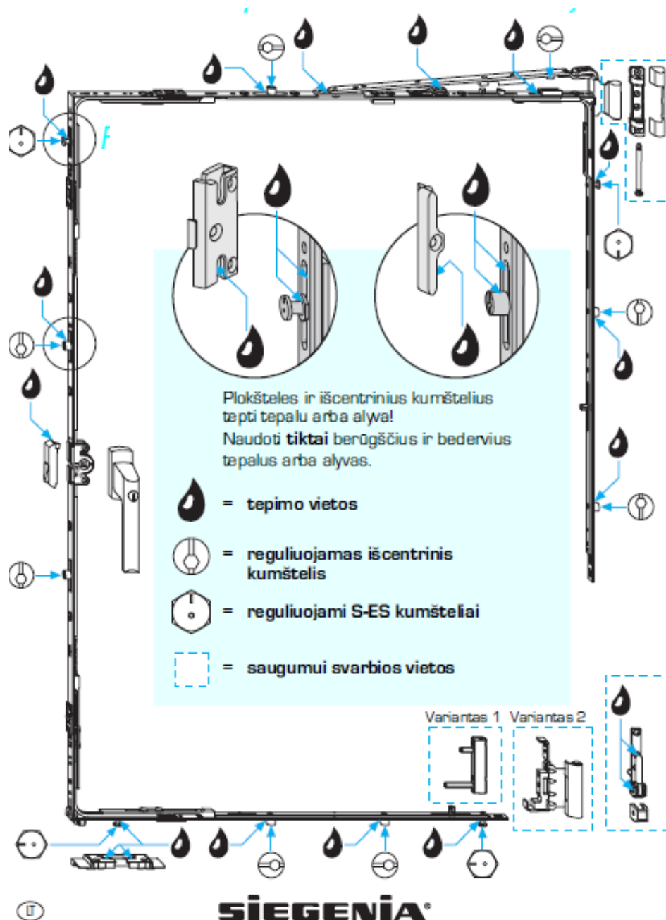
Pav. 1 Principinė langų apkaustų priežiūros schema
